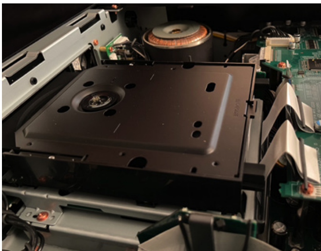
Audiooptimiertes Laufwerk für CD und SACD
